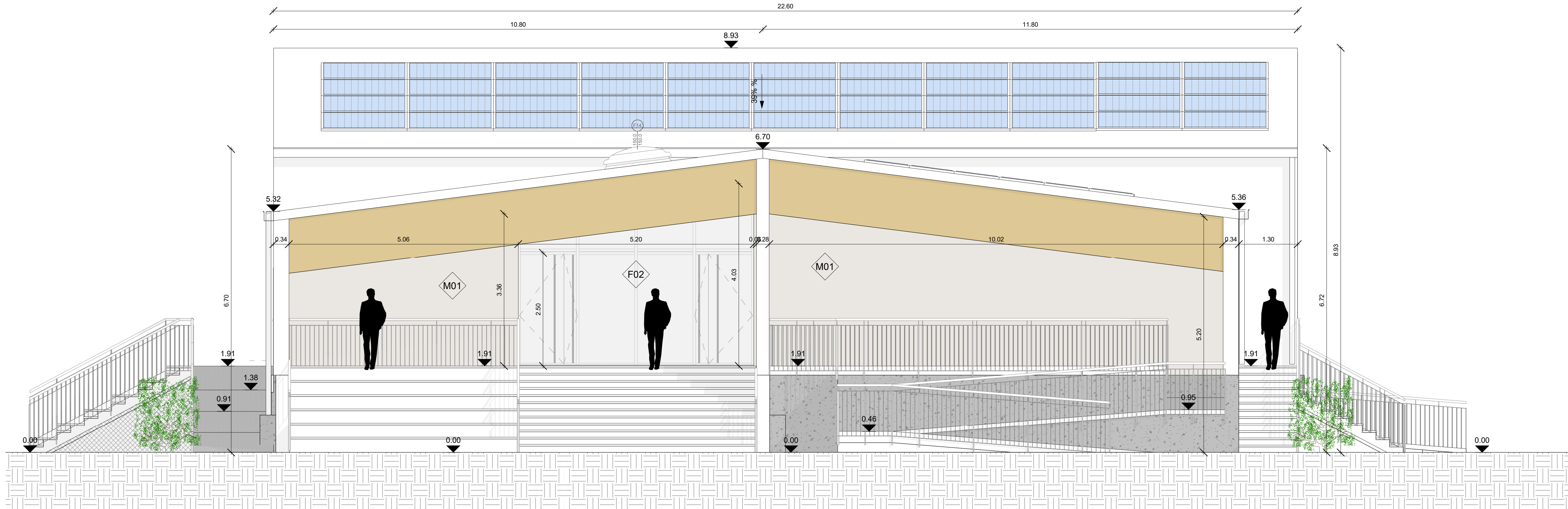
② Prospetto Sud 1 : 50
