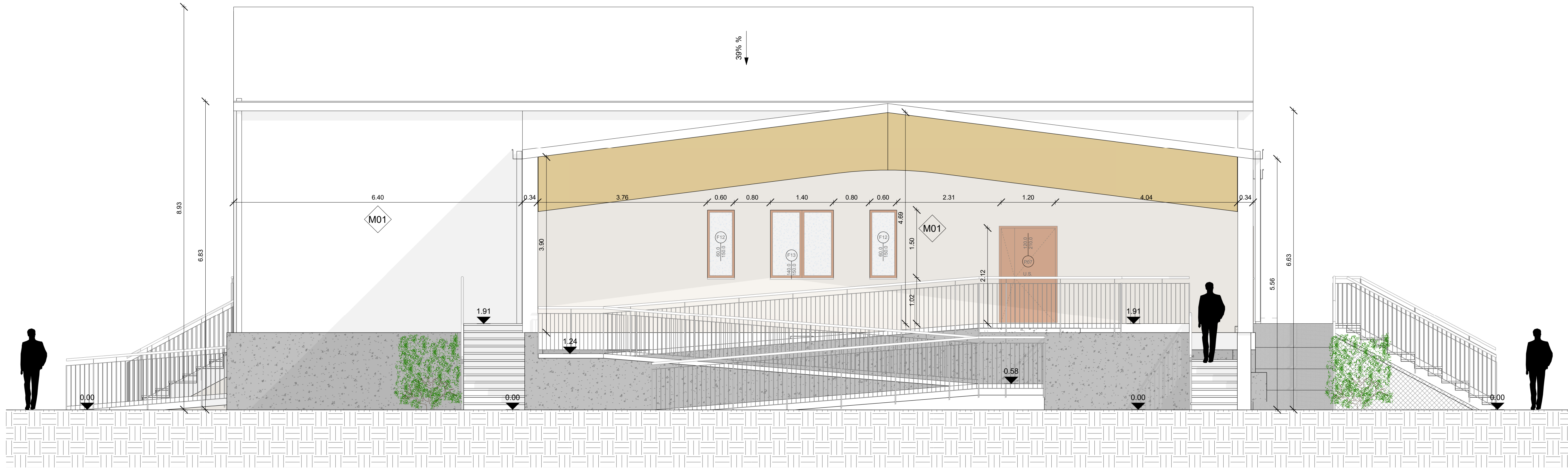
② Prospetto Sud 1 : 50
