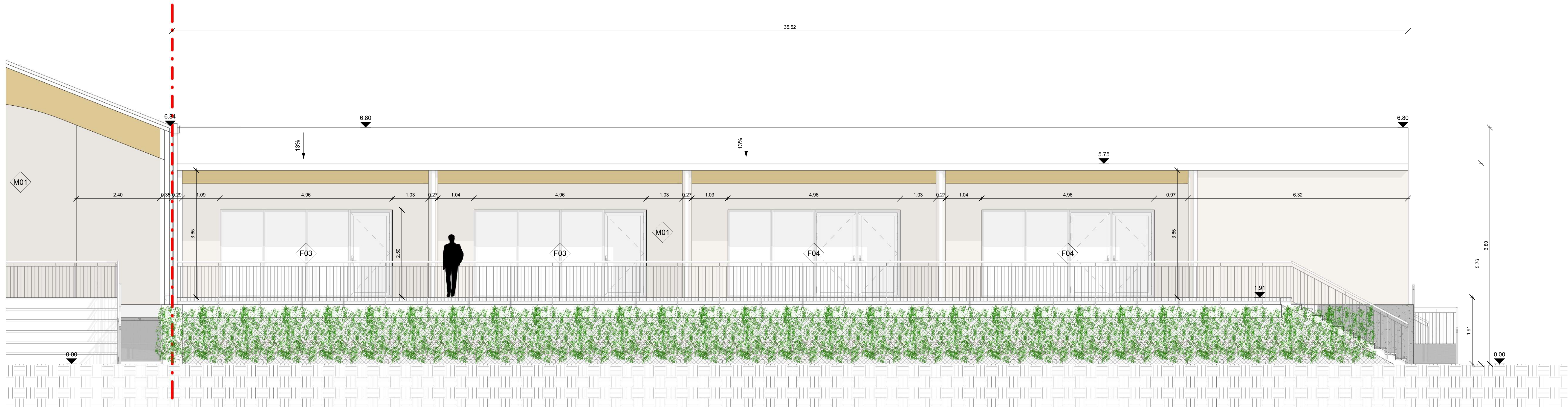
3 Prospetto Ovest -Stralcio 03 1 : 50
