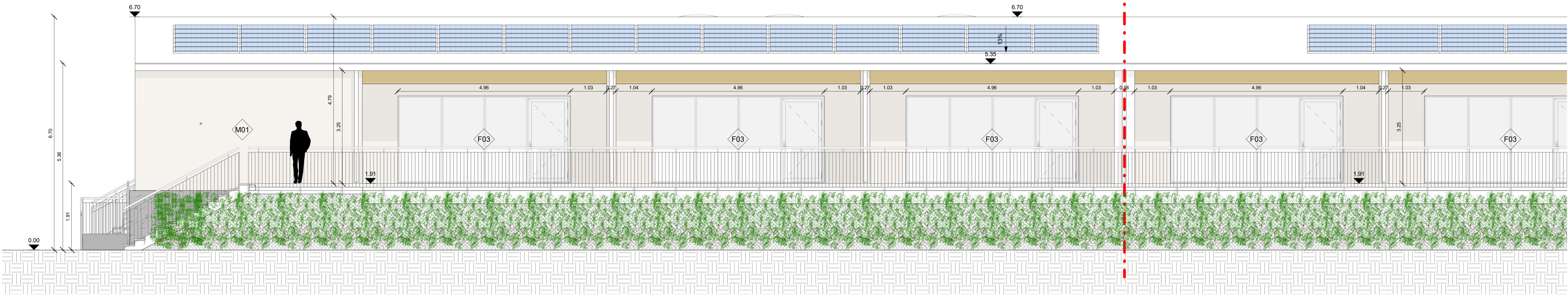
2 Prospetto Ovest - Stralcio 02 1 : 50
